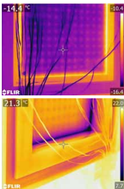
Termovízna snímka okna v klíma komore
