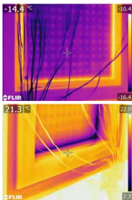
Termovízna snímka okna v klíma komore
