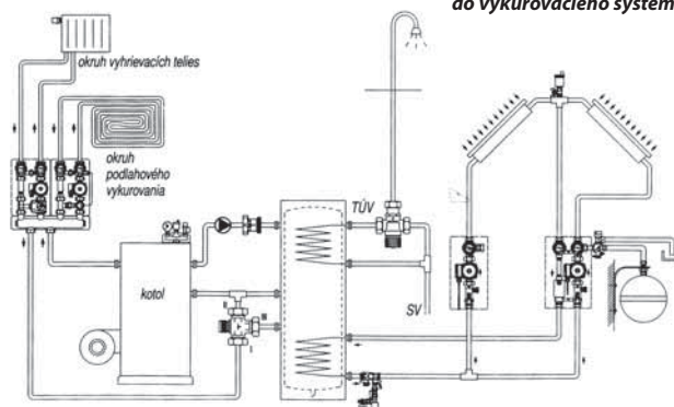
Príklad integrácie solárnej sústavy do vykurovacieho systému:
