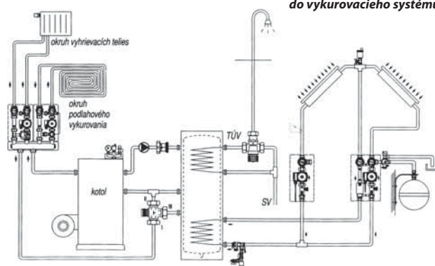
Priklad integrácie solárnej sústavy do vykurovacieho systému:
