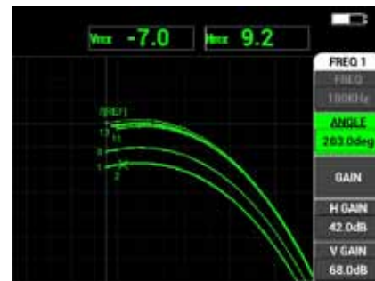
Signál vírivých prúdov od vybraných vzoriek
