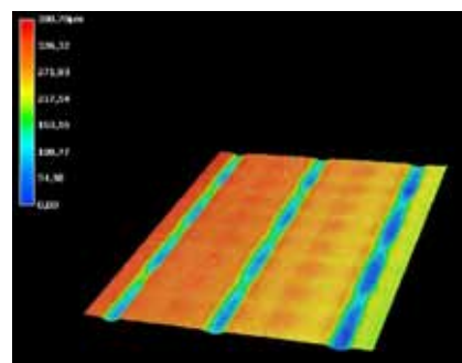
Stanovenie plochy priečného rezu drážkou pre Monel 400 – kombinácia faktorov 5
