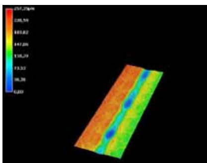
Topografická mapa drážky (Monel 400 vľavo, Titán GR5 vpravo)
