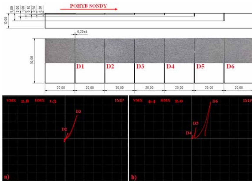
Signálové krivky od rôznych veľkostí defektu
