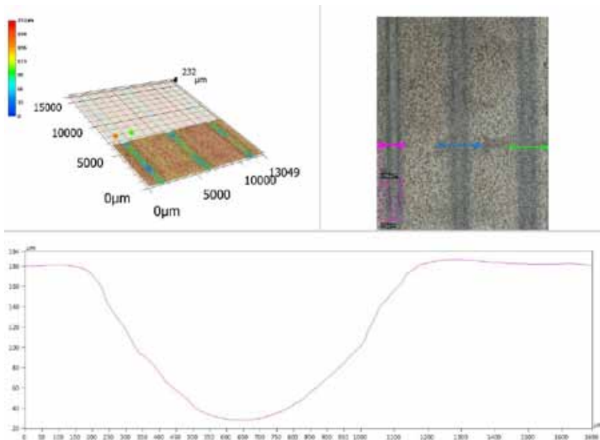
Porovnanie drážok (konštantné \alpha a m , so zmenou uhla naklonenia) Ti GR5
