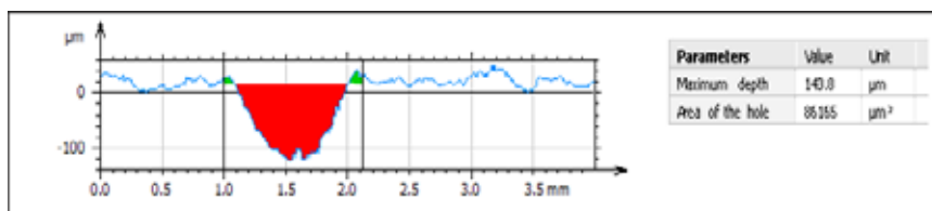
Stanovenie plochy priečného rezu drážkou pre Monel 400 – kombinácia faktorov 5
